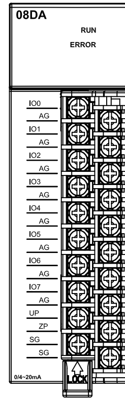
AH08DA-5C
