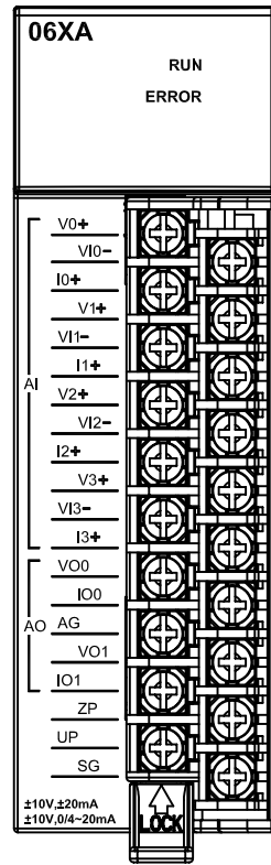
AH06XA-5A
