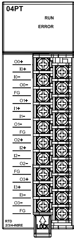
AH04PT-5A
