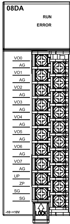
AH08DA-5B
